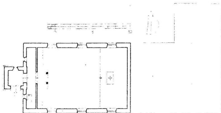
Fig. 2 KEEKEN, ev. Kirche. Grundriß 1:300
